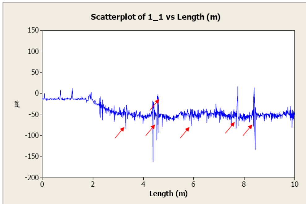
Figura 6. Calibraciones de la fibra óptica.
