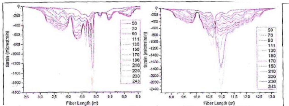
Figura 3. Longitudes de las deformaciones en la fibra (primer y segundo tramo).
